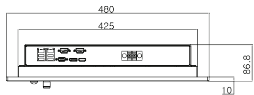
BOTTOM VIEW(DC)
