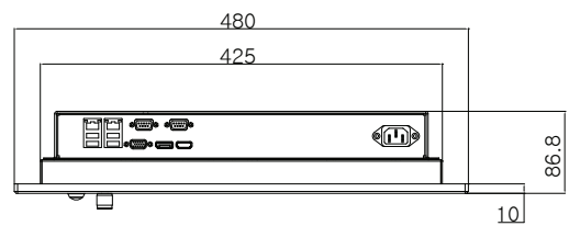
BOTTOM VIEW(AC)
