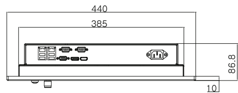
BOTTOM VIEW(AC)
