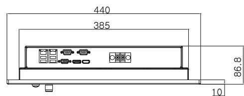
BOTTOM VIEW(DC)
